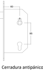
Cerradura antipánico
