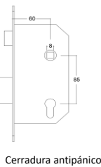
Cerradura antipánico
